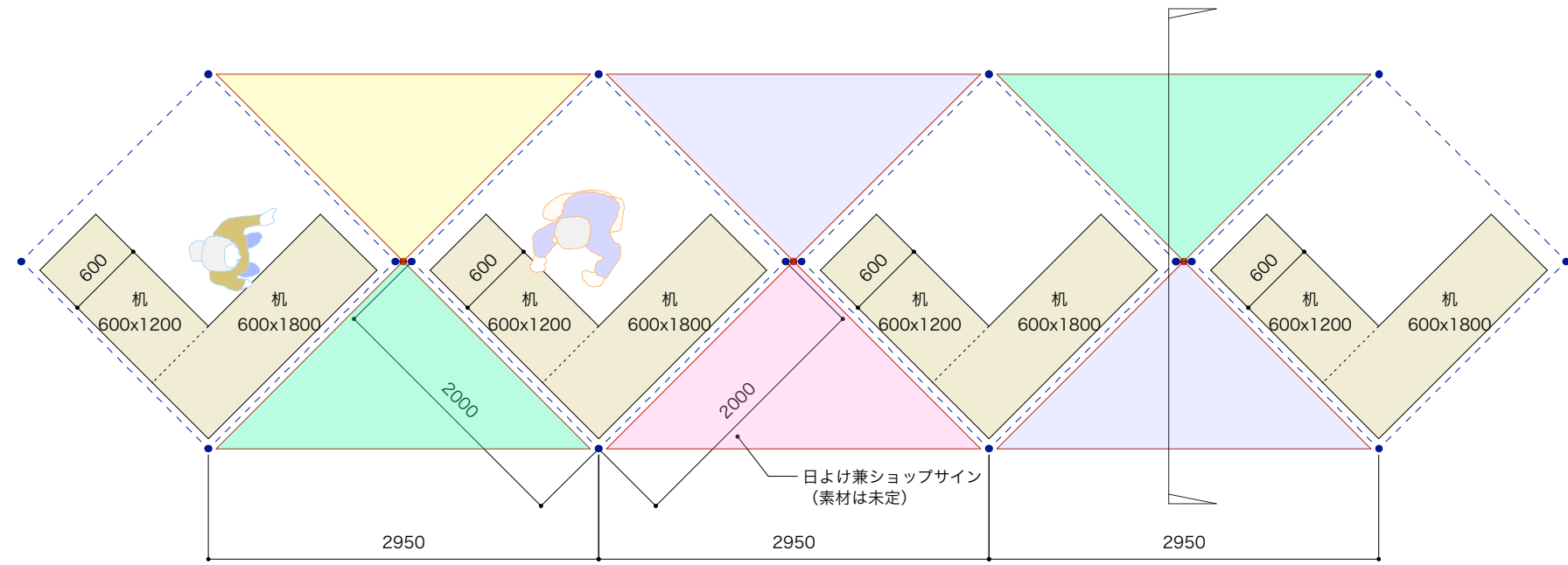
plan S=1/50 ※机はオプション
